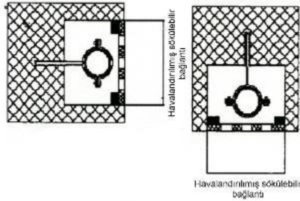
Şekil 9 — Duvar/Asma tavan içi kanal ve boru geçiş detayı
