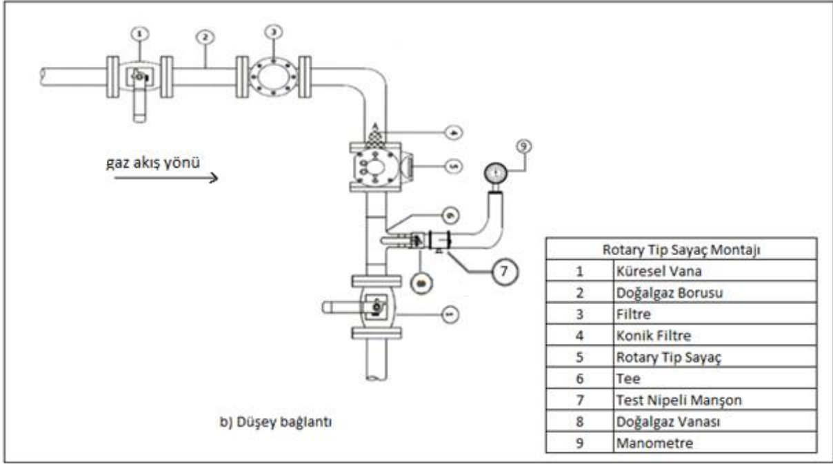
Şekil 15 — Rotary sayaçlara ait bağlantı detayı
