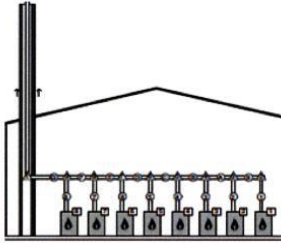
Şekil 24 — Kaskad baca sistemi
