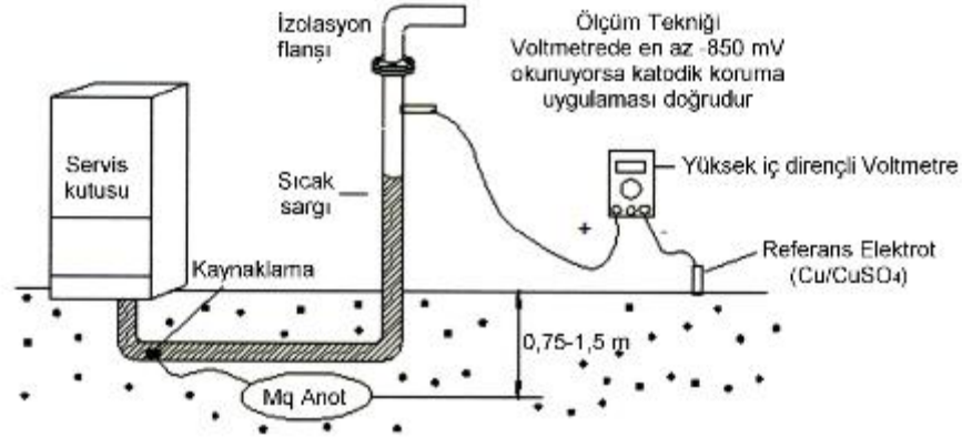
Şekil 6 – Katodik Koruma
