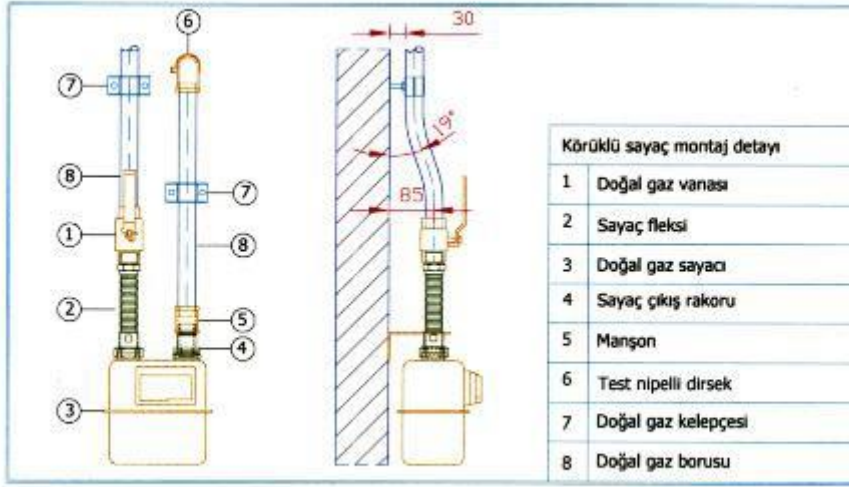
Şekil – 12 Körüklü Sayaç bağlantı detayı
