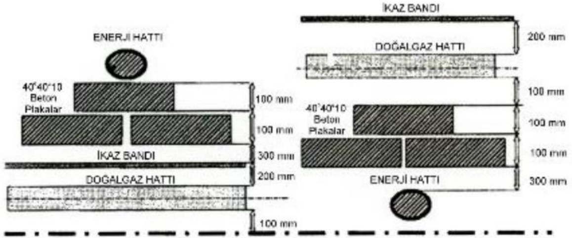
Şekil - 3 Doğal gaz hattı ile elektrik kabloları arasındaki mesafe
