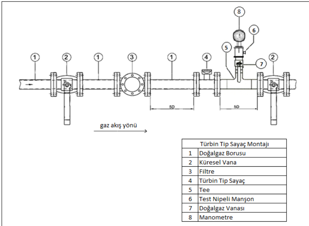
Şekil 16 — Türbinli sayaçlara ait bağlantı detayı
