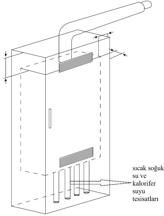
Şekil – 20 kabin detayı
