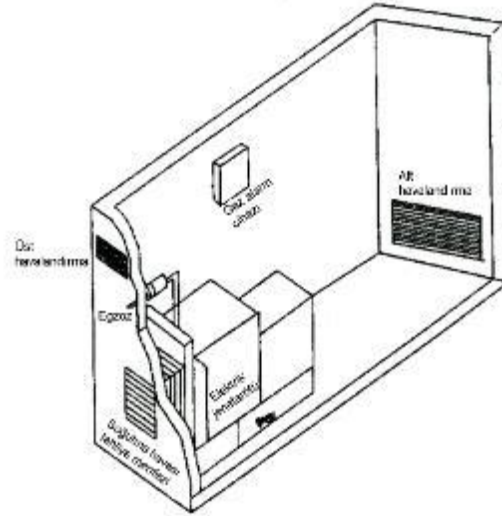
Şekil 25 — Elektrik jeneratör dairesi
