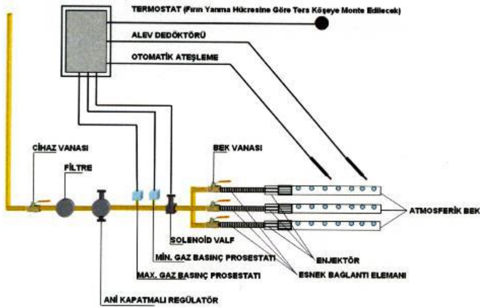
Şekil 26 — Fırınlarda brülör emniyet ekipmanları montaj şeması
